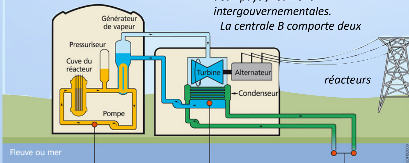
Circuit primaire
